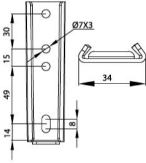
M02010250 Ürün No/Prod. No: 76 KOL KAVRAMA KIZAĞI (12 cm) SLIDING HINGE (12 cm)
