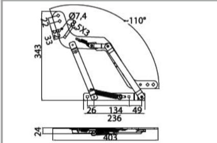
M02010292 Ürün No/Prod. No: 70 BALKAN MEKANİZMASI (KÜÇÜK KISA KOLLU) BALKAN MECHANISM (SMALL SHORT ARMED)
