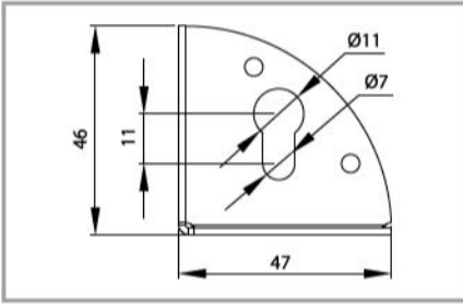
M02010242 Ürün No/Prod. No: 83 BAZA KULBU MENTEŞESİ BASE HANDLE HINGE
