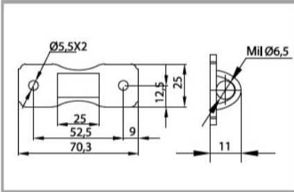
M02010242 Ürün No/Prod. No: 83 BAZA KULBU MENTEŞESİ BASE HANDLE HINGE
