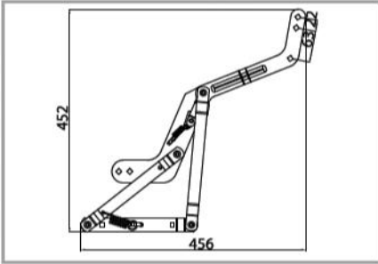
M02010292 Ürün No/Prod. No: 70 BALKAN MEKANİZMASI (KÜÇÜK KISA KOLLU) BALKAN MECHANISM (SMALL SHORT ARMED)
