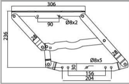
M02010122 Ürün No/Prod. No: 63 KÖŞE MEKANİZMASI (KÜÇÜK) CORNER MECHANISM (SMALL)
