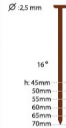
45mm Ürün No/Prod.No:200.1 50mm Ürün No/Prod.No:200.2 55mm Ürün No/Prod.No:200.3 60mm Ürün No/Prod.No:200.4 65mm Ürün No/Prod.No:200.5 70mm Ürün No/Prod.No:200.6
